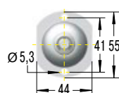
PG5-V4A Rundbeslag
