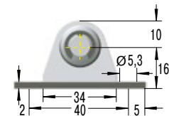
NA5-V4A Winkelbeslag
