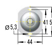
PA5-V4A Rundbeslag
