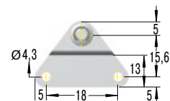
OG5-V4A Seitenbeslag
