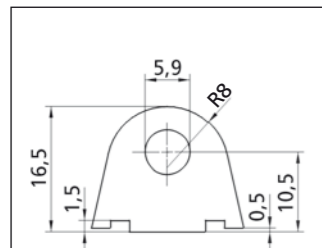
Tiefe: 15 mm Profil-Nr. 2.3.3.016.020
