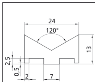
Tiefe: 15 mm Profil-Nr. 2.3.3.013.024
