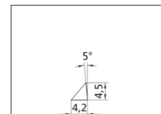
Profil-Nr. 2.3.2.018.020
