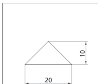
Tiefe: 100 mm Profil-Nr. 2.3.3.020.010
