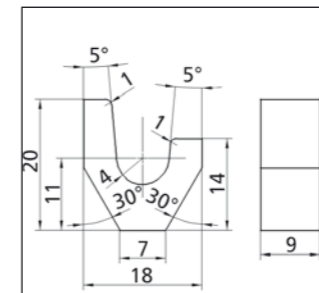
Profil-Nr. 2.3.2.018.020
