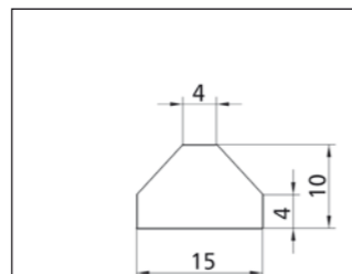
Tiefe: 25 mm Profil-Nr. 2.3.3.004.005
