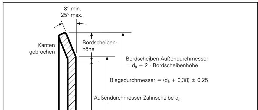
Bordscheibe
