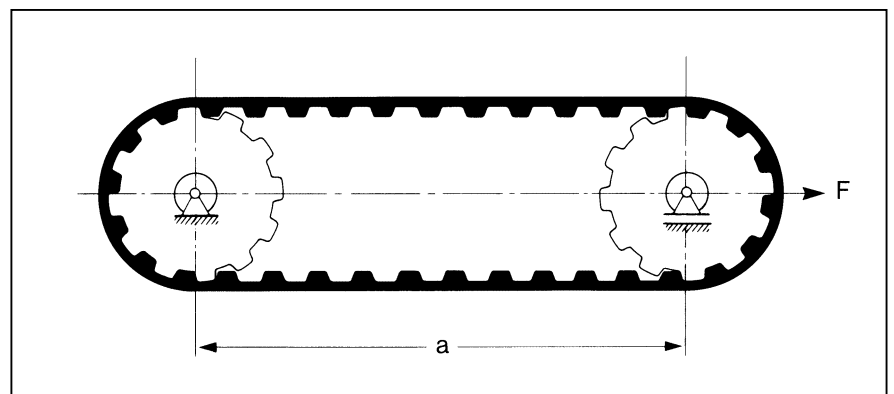
Meßanordnung
