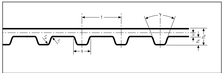
Zahnriemenprofil
